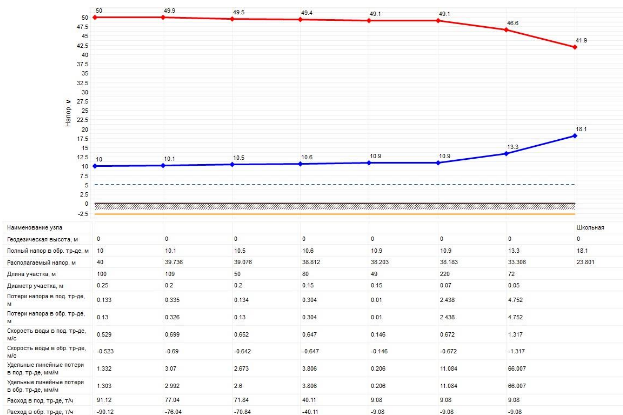
Рисунок 2.45 – Пьезометрический график от Котельной п. Нагорный до самого удаленного потребителя в аварийной ситуации по ул. Школьная
