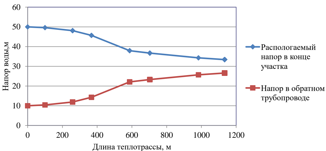
Рисунок 2.11 – Пьезометрический график тепловой сети Котельная п. Нагорный до ул. Молодежная
