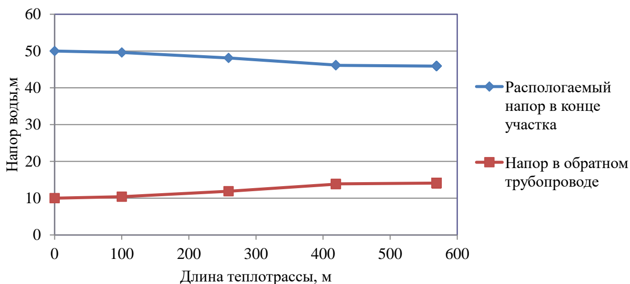
Рисунок 2.15 – Пьезометрический график тепловой сети Котельная п. Нагорный до ул. Боровая, 9
