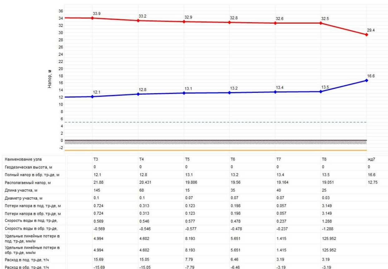
Рисунок 2.46 – Пьезометрический график от источника теплоснабжения (Котельной п. Синий Бор) до самого удаленного потребителя в аварийной ситуации
