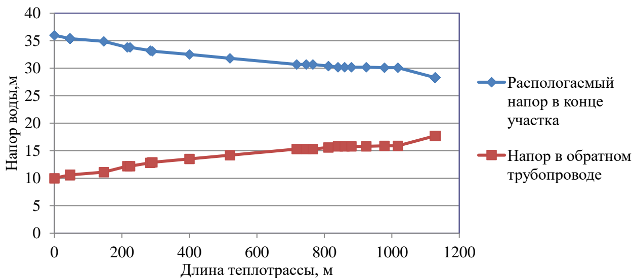
Рисунок 2.19 – Пьезометрический график тепловой сети Котельной №2 с. Кичигино до домов по ул. Комсомольская
