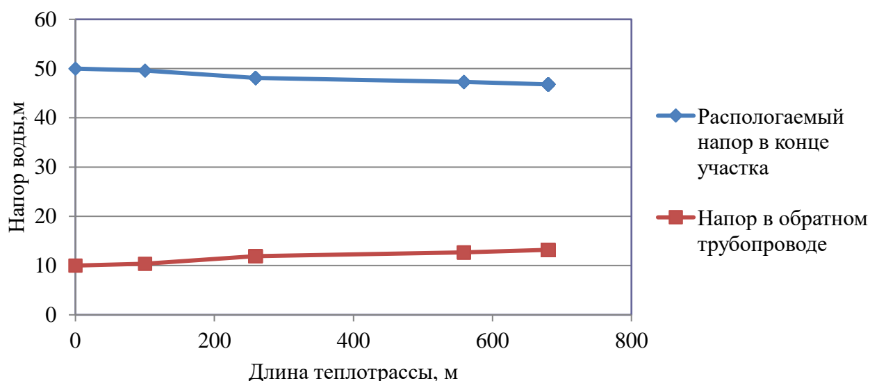
Рисунок 2.13 – Пьезометрический график тепловой сети Котельная п. Нагорный до ул. Садовая, 17
