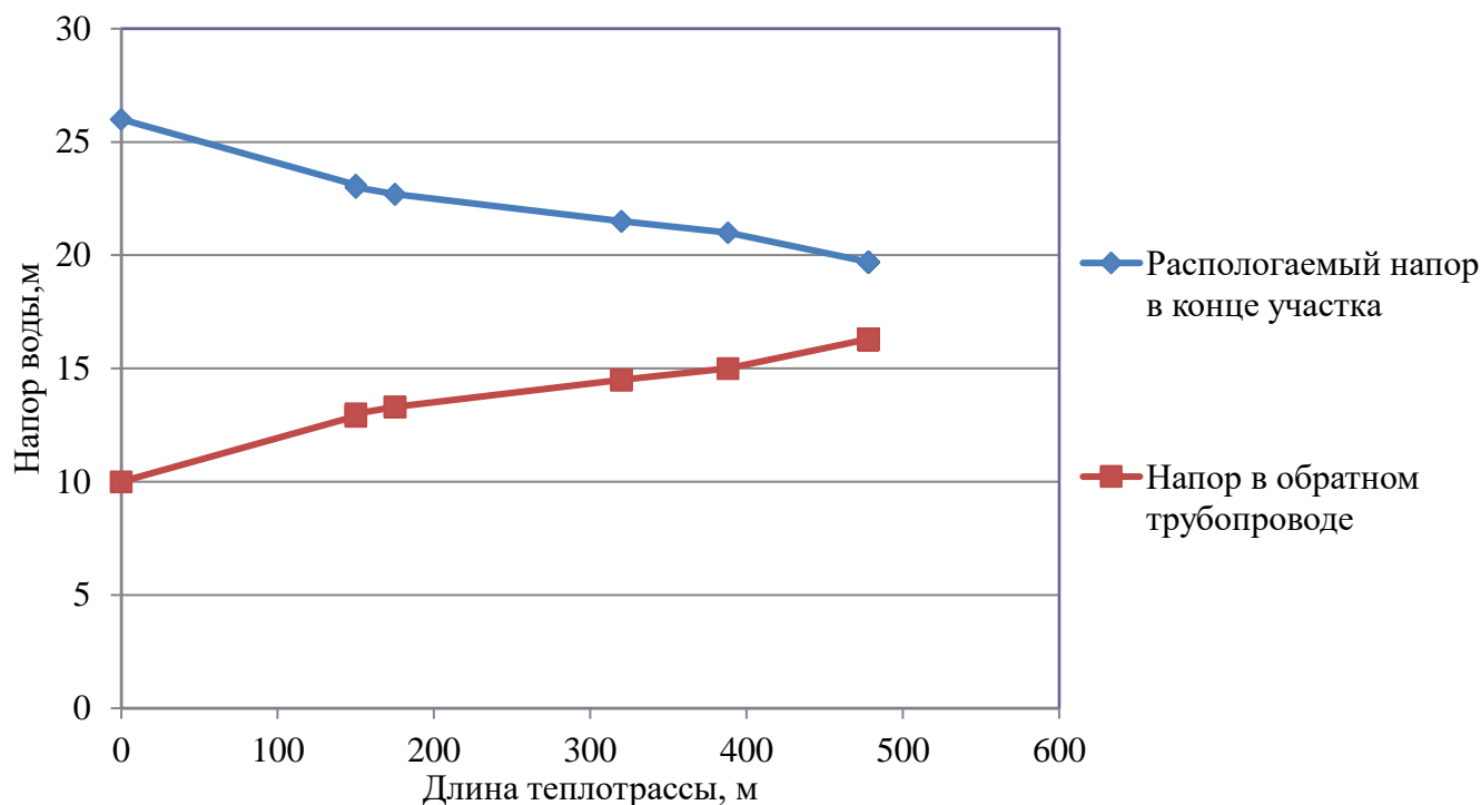
Рисунок 2.16 – Пьезометрический график тепловой сети Котельная п. Синий Бор
