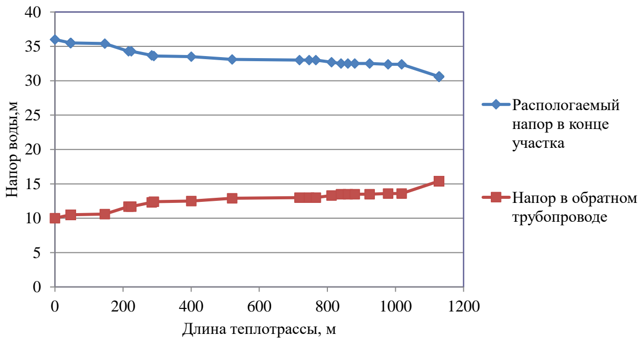
Рисунок 2.9 – Пьезометрический график тепловой сети Котельная №2 с. Кичигино до частных домов по ул. Комсомольская
