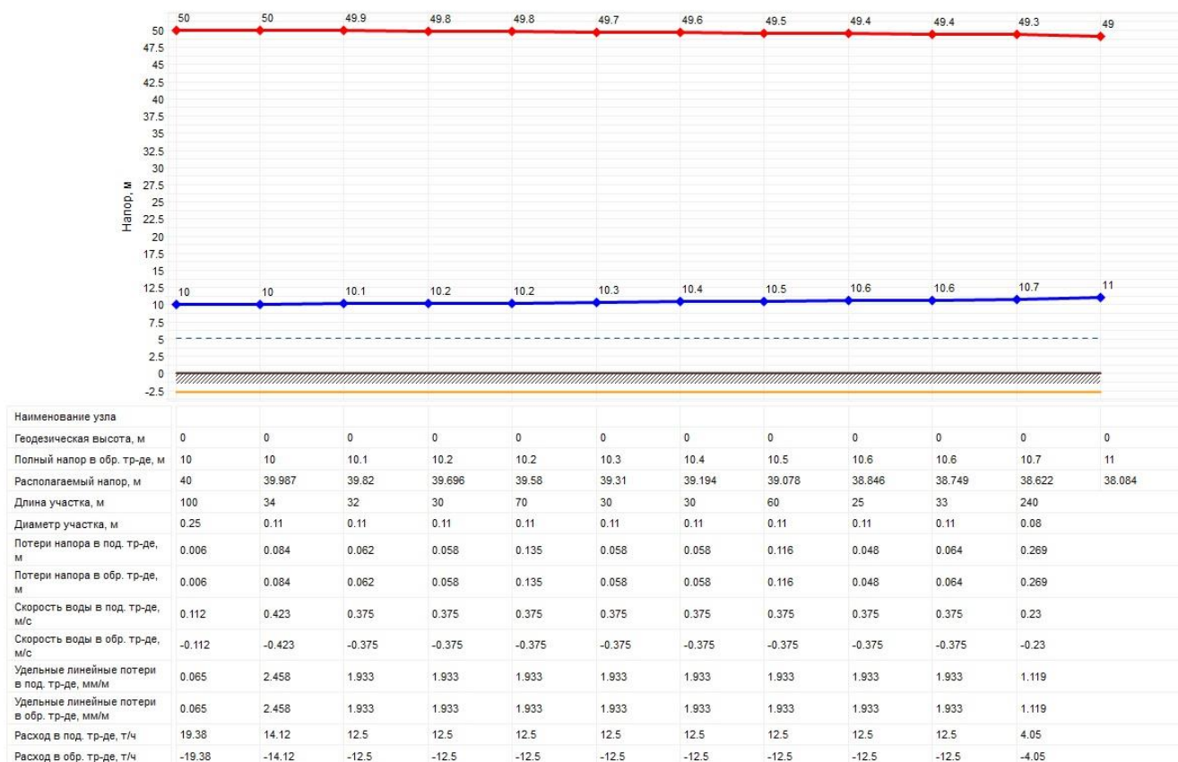
Рисунок 2.35 – Пьезометрический график от источника теплоснабжения (Котельной п. Нагорный) до самого удаленного потребителя – детского сада
