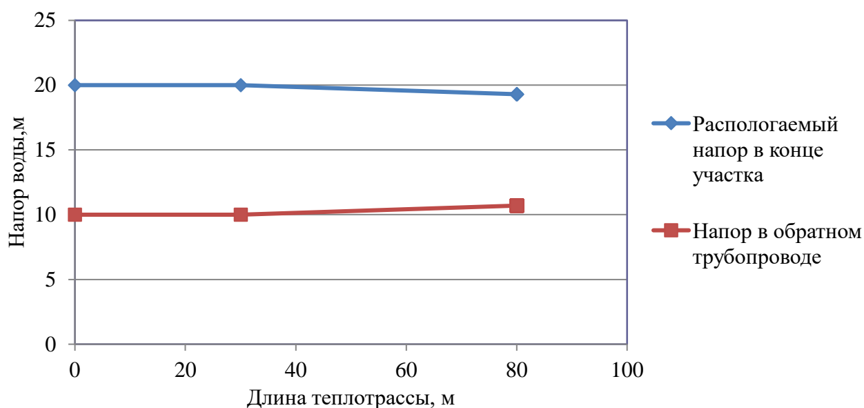
Рисунок 2.20 – Пьезометрический график тепловой сети Котельная ТКУ-1000 с. Кичигино
