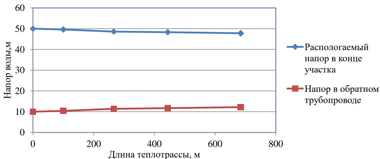
Рисунок 2.22 – Пьезометрический график тепловой сети Котельная п. Нагорный до детского сада
