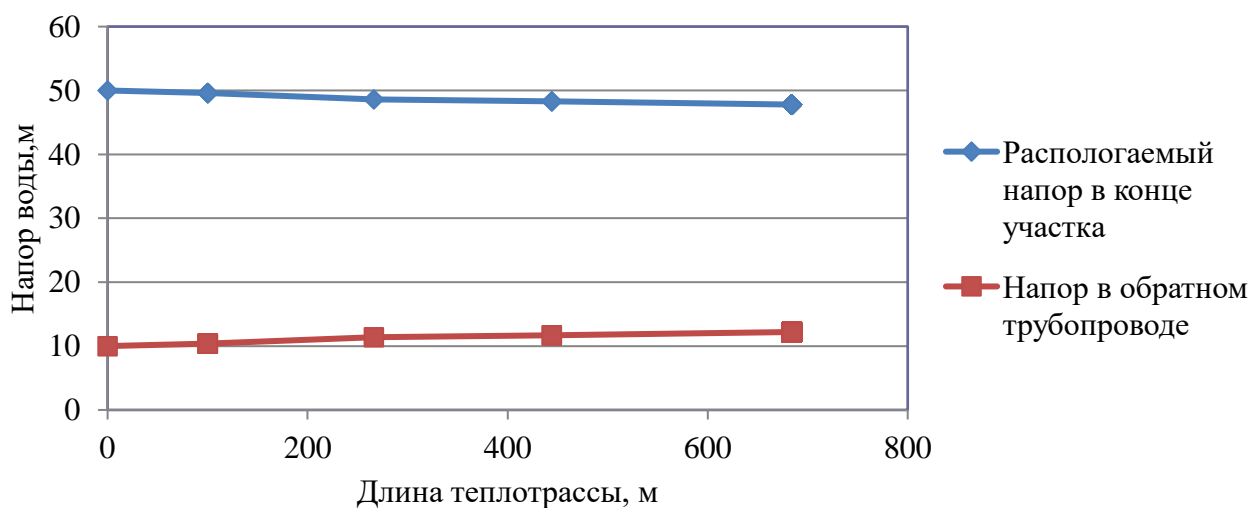
Рисунок 2.12 – Пьезометрический график тепловой сети Котельная п. Нагорный до детского сада
