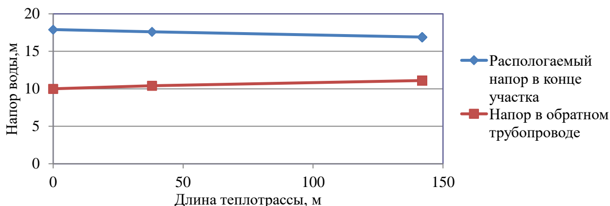
Рисунок 2.7 – Пьезометрический график тепловой сети Котельной №1 с. Кичигино
