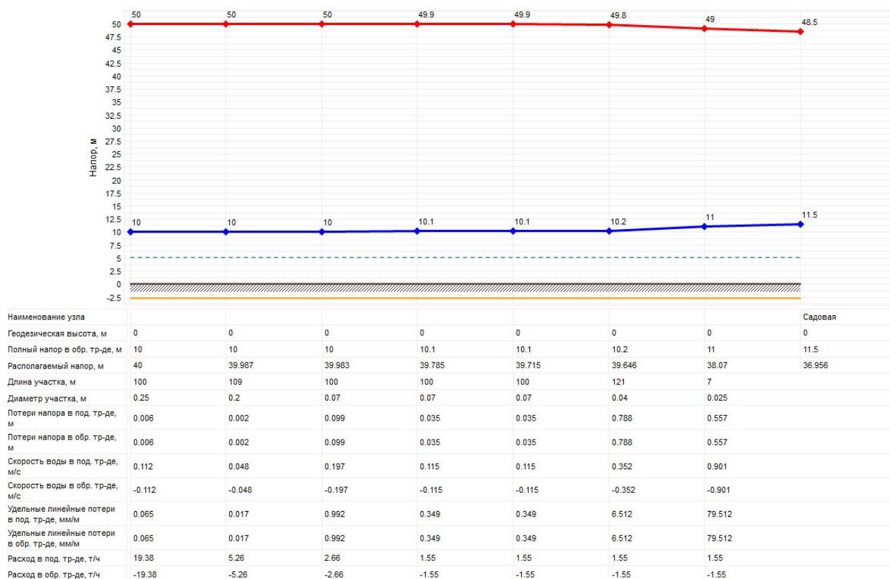
Рисунок 2.34 – Пьезометрический график от источника теплоснабжения (Котельной п. Нагорный) до самого удаленного потребителя по ул. Садовая
