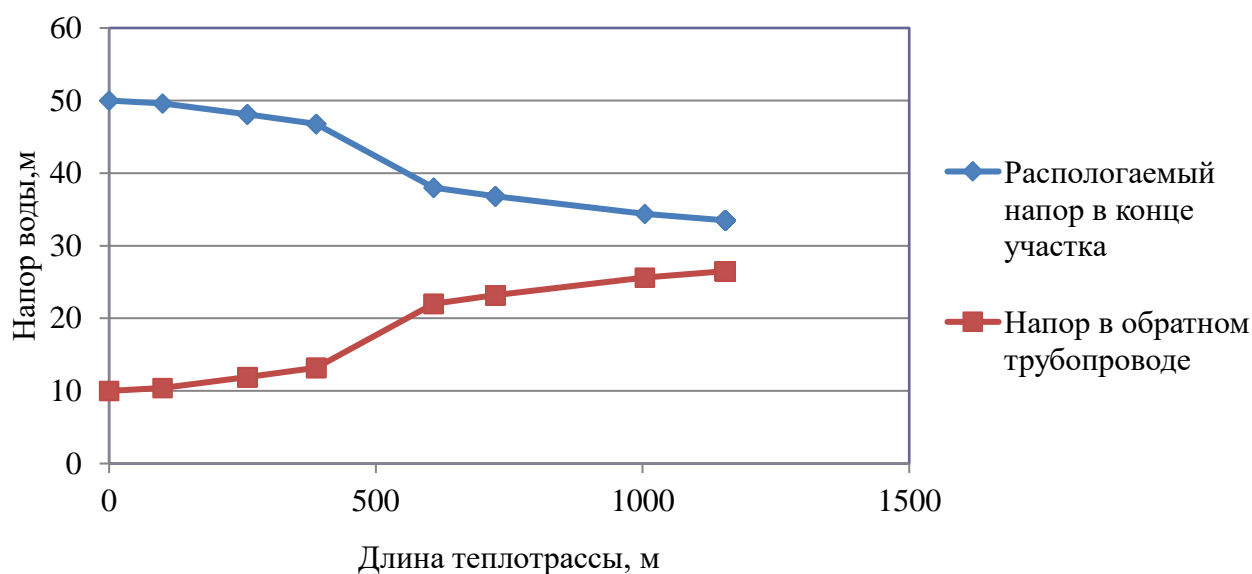
Рисунок 2.21 – Пьезометрический график тепловой сети Котельная п. Нагорный до ул. Молодежная
