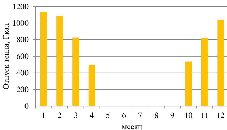
Рисунок 1.6 Оптимальный температурный график отпуски тепловой энергии для Котельная №2 с. Кичигино с температурным режимом 85-64 °С
