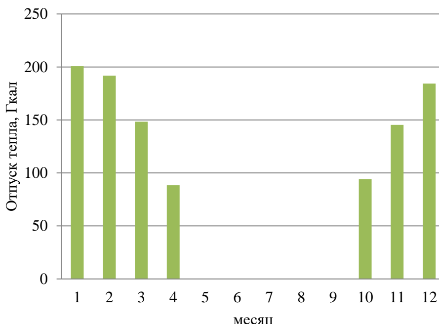
Рисунок 1.9 Оптимальный температурный график отпуска тепловой энергии для Котельная п. Синий Бор с температурным режимом 90-70 °С
