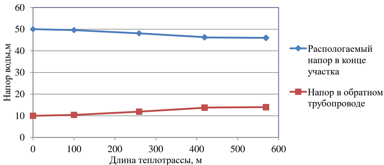
Рисунок 2.25 – Пьезометрический график тепловой сети Котельная п. Нагорный до ул. Боровая
