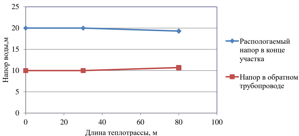
Рисунок 2.10 – Пьезометрический график тепловой сети Котельная ТКУ-1000 с. Кичигино
