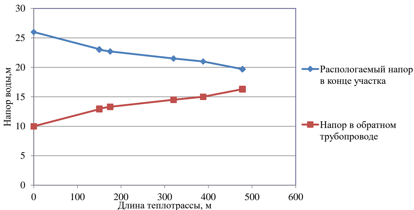
Рисунок 2.26 – Пьезометрический график тепловой сети Котельная п. Синий Бор
