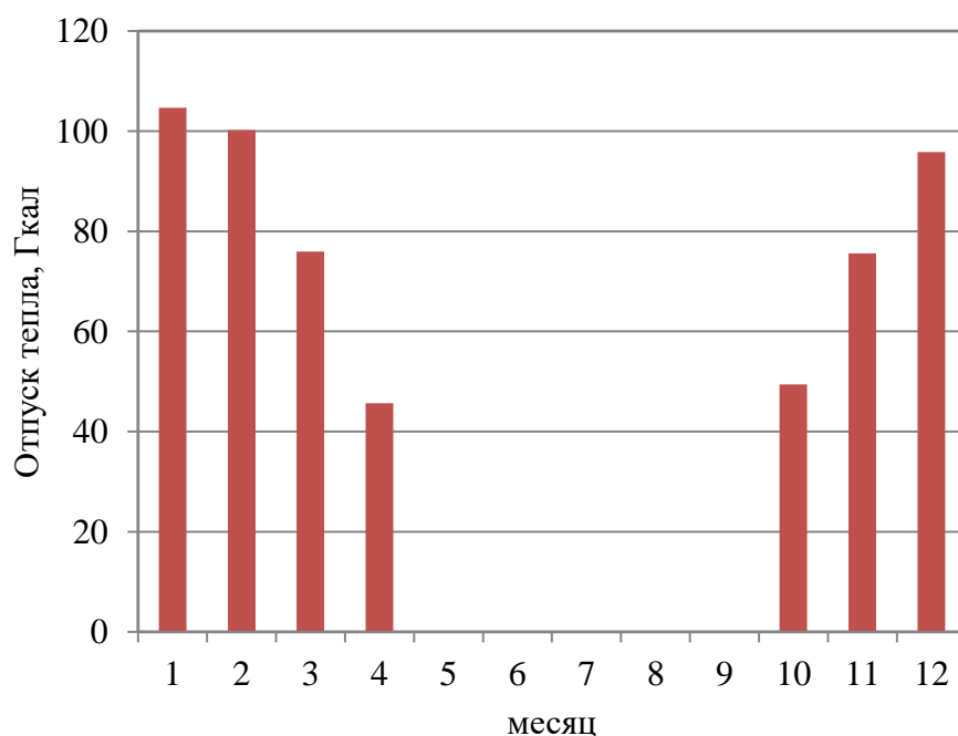
Рисунок 1.5 – Оптимальный температурный график отпуска тепловой энергии для Котельной №1 с. Кичигино с температурным режимом 85-64 °С
