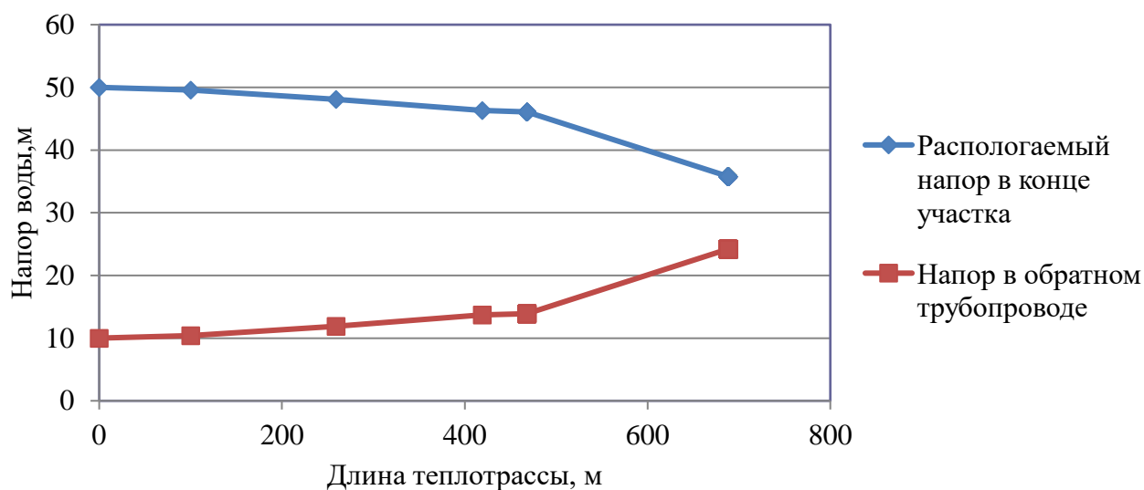
Рисунок 2.14 – Пьезометрический график тепловой сети Котельная п. Нагорный до ул. Школьная, 8
