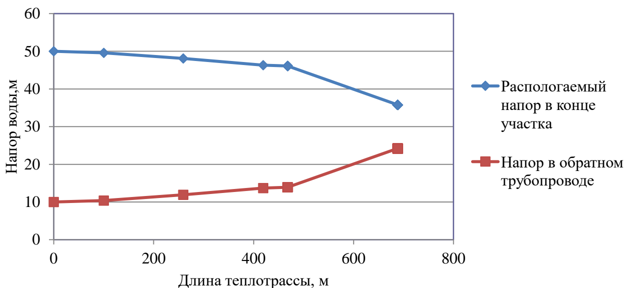
Рисунок 2.24 – Пьезометрический график тепловой сети Котельная п. Нагорный до ул. Школьная
