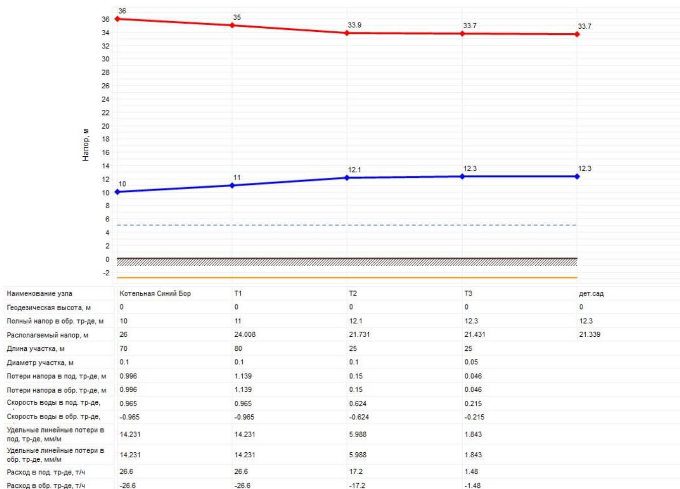
Рисунок 2.36 – Пьезометрический график от источника теплоснабжения (Котельной п. Синий Бор) до самого удаленного потребителя
