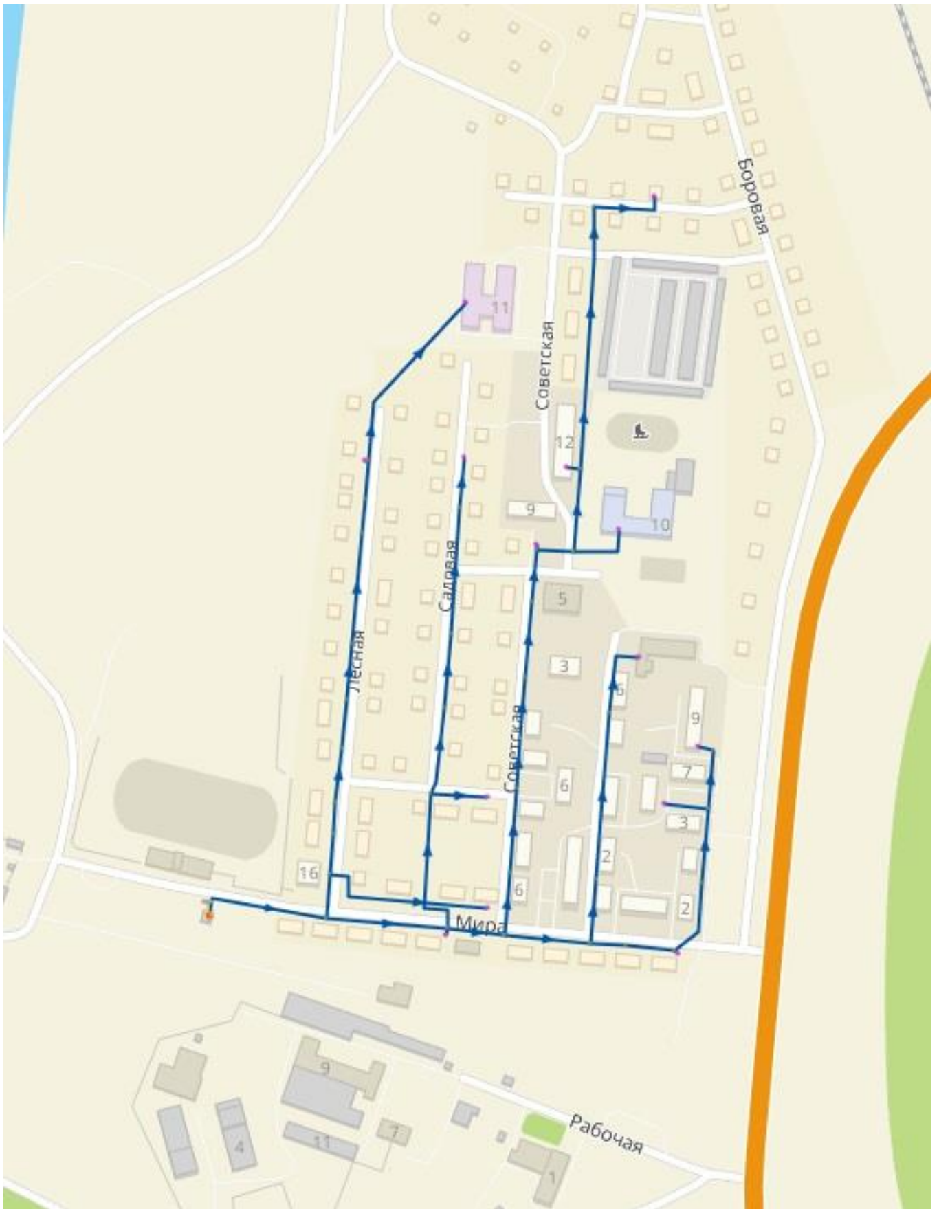
Рисунок 2.31 – Модель системы теплоснабжения Котельной п. Нагорный
